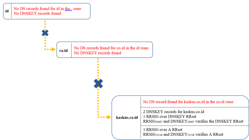
Figure 14: kaskus.co.id
